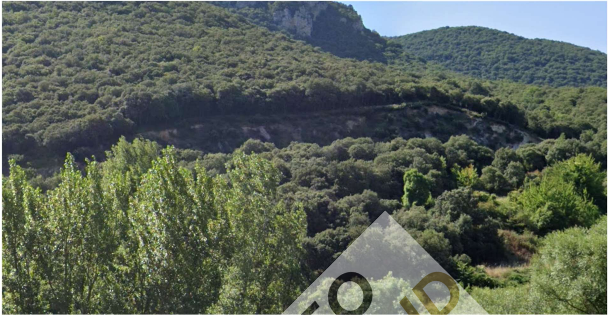
Panorámica del talud antes de la instalación de geomalla, red de cable y bulones.
