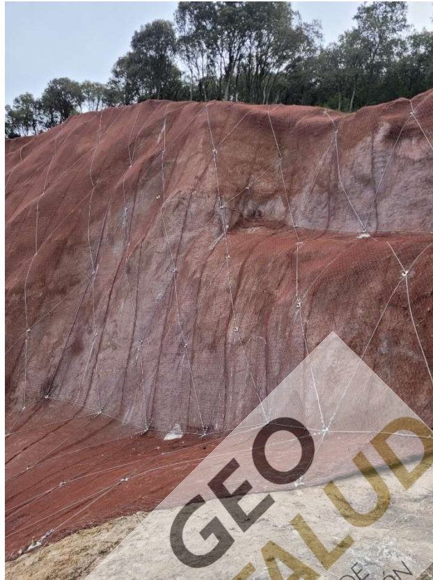
Detalle del refuerzo y adaptado al talud mediante cable y bulones.
