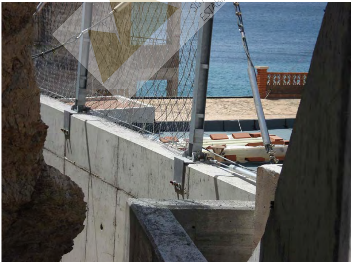
Detalles barrera con capacidad de absorción de energía de 250 KJ y H = 3m, colocada sobre muro de hormigón
